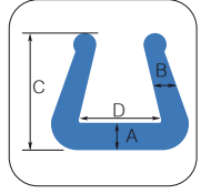
U PROFİL
